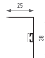
GUÍA LATERAL CIERRE-IMÁN
